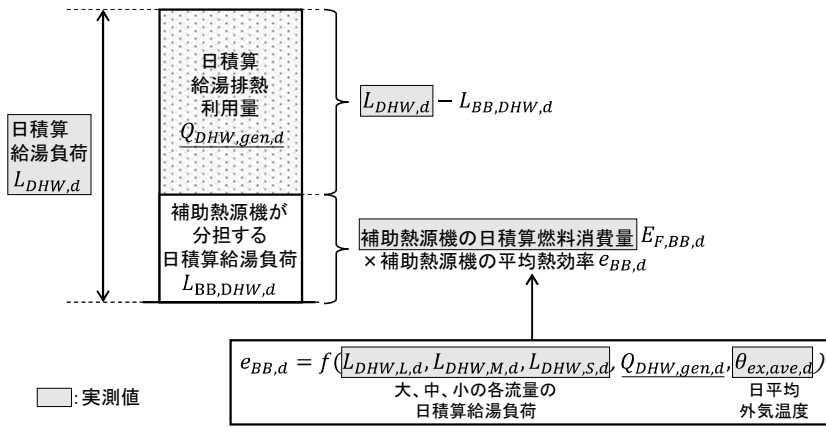
図4 日積算給湯排熱利用量 Q_{DHW,gen,d} の概念図
